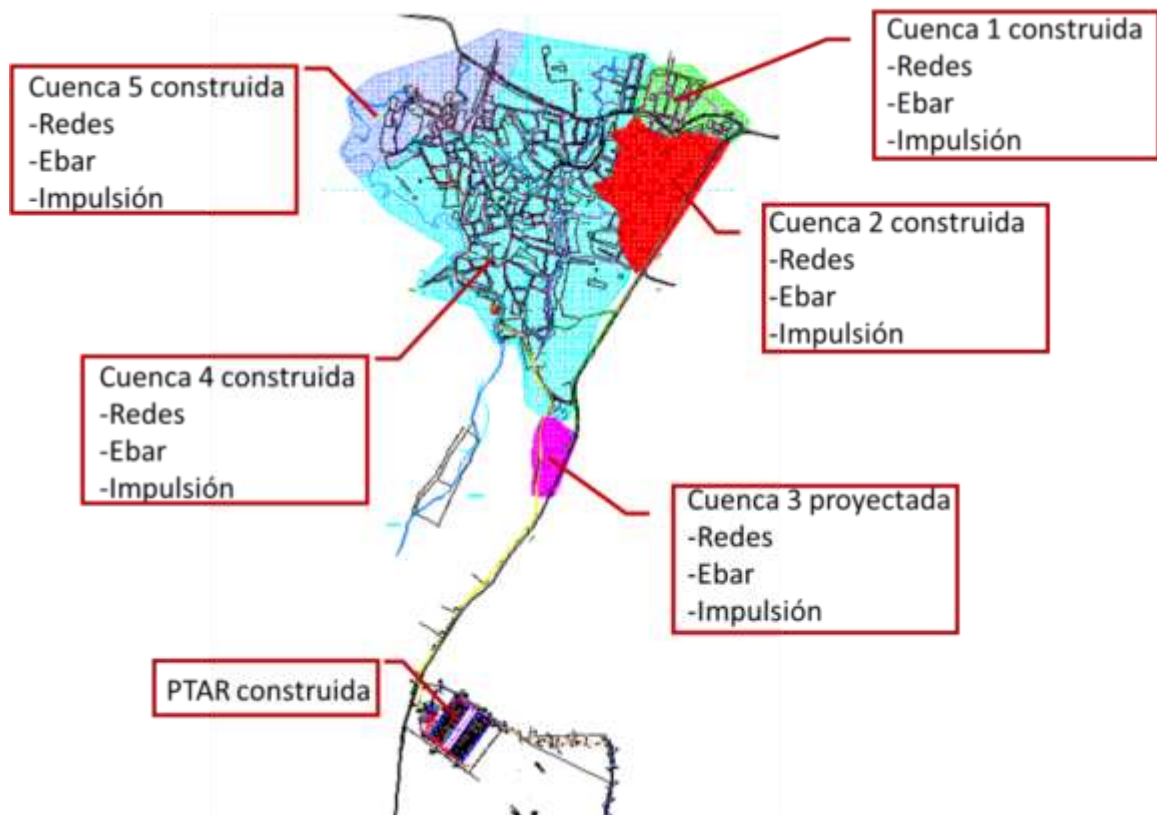
Imagen 2. Integralidad Sistema de Alcantarillado Municipio de Usiacurí.
