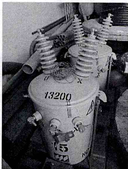
Suministro de dos transformadores monofásicos
