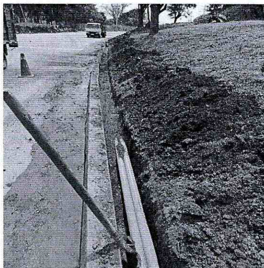
Instalación de Tubería PVC DB de 2"
