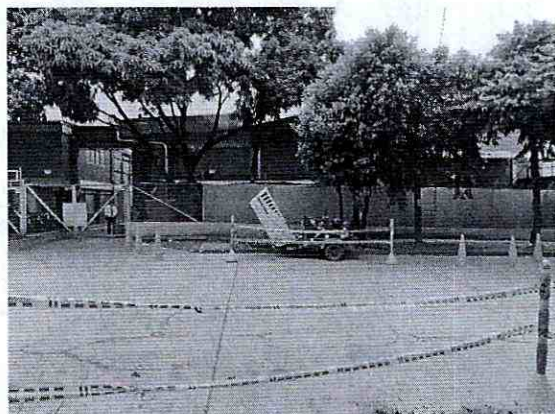
Canalizacion de tuberia pvc 2" en calzada, excavacion con compresor de bala teledirigida de 5" (topo)
