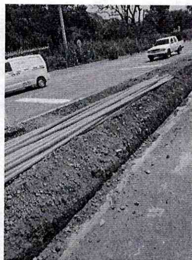
Instalación de Tubería PVC DB de 2"
