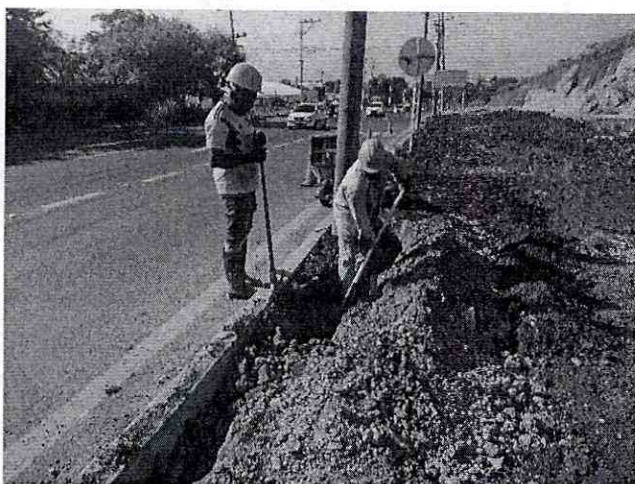
Excavación manual sin retiro
