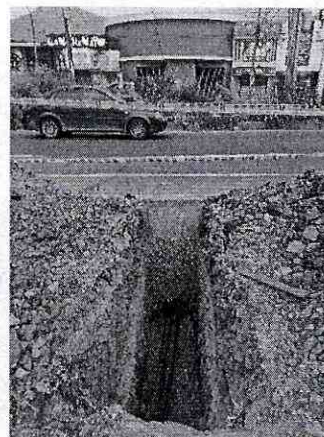
Canalización de tubería pvc 2" en calzada, excavación con compresor de bala teledirigida de 5" (topo)
