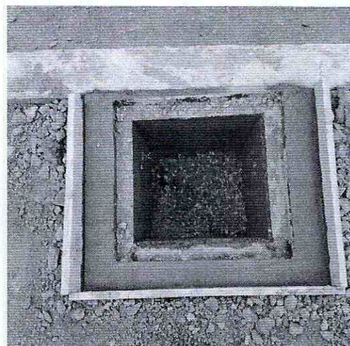
Construcción cámaras de registro norma Emcali (40x40x75 cms).
