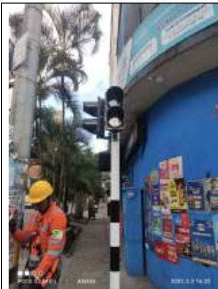
Fotografía 14: Instalación semáforo. Carrera 43 con calle 55
