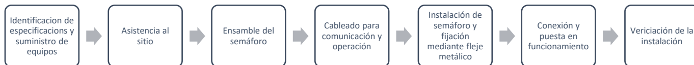
Gráfico 3: Proceso en la instalación de semáforo vehicular
