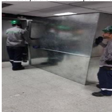
Imagen N° 4. Pesaje de Ducteria en Lámina Galvanizada para Uma N 1 del piso 7 – CAD.
