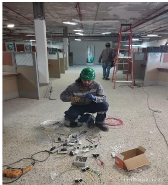
Imagen N° 47. Instalación de red de iluminación Sótano A.
