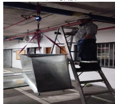
Imagen N° 10. Ajustes CVV Piso 7 – CAD.
