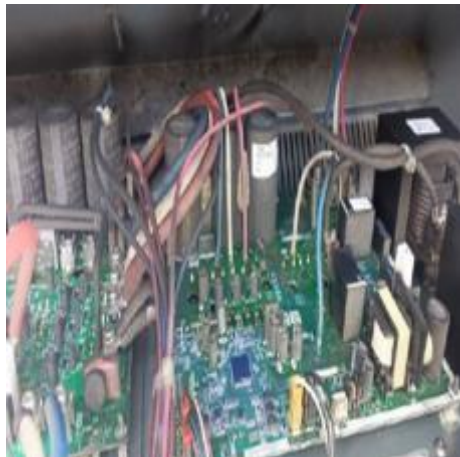
Imagen N° 17. Inspección y diagnostico sistema VRV Daikin..
