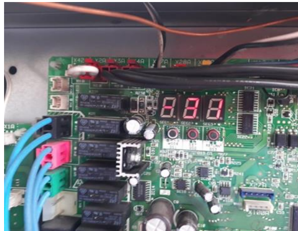
Imagen N° 4. Revisión de Equipos VRV Secretaría de Movilidad.
