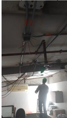
Imagen N° 71. Instalación salidas de iluminación taquillas de espectáculos.
