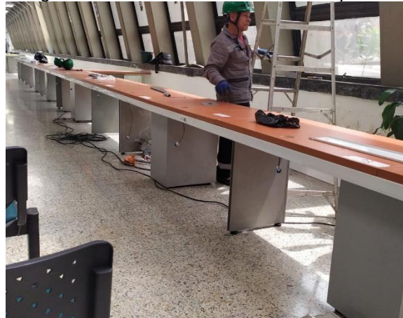
Imagen N°40. Desinstalación redes eléctricas sótano A.
