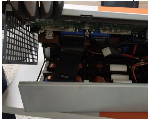
Imagen N° 2247. Mantenimiento UPS piso 3.
