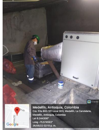
Imagen N° 12. Revisión de equipo UMA auditorio Plaza Libertad.
