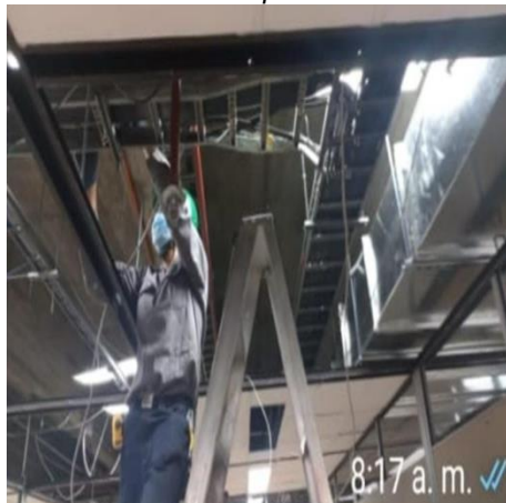
Imagen N° 3. Suministro lámina galvanizada Uma Tecam 1 - piso 7.
