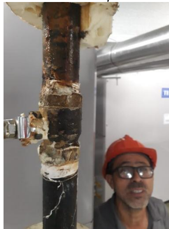
Imagen N° 18. Revisión y diagnóstico de válvula en cuarto técnico piso 13
