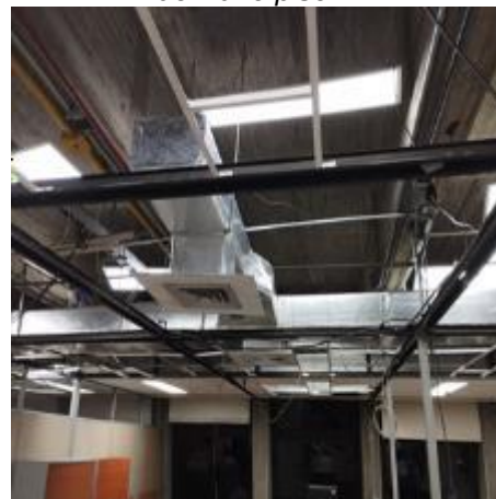
Imagen N° 8. Desmonte de ducteria en lámina fibra de vidrio piso 7.
