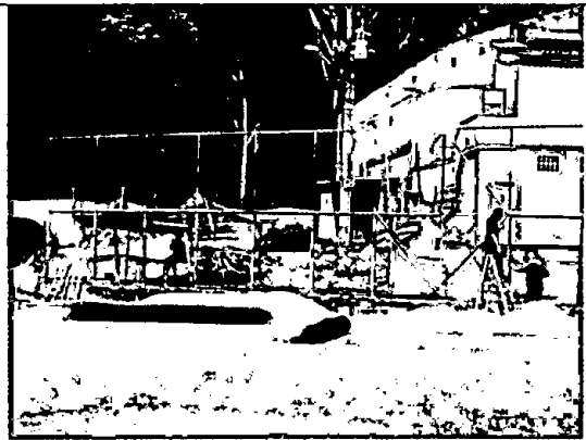
Fotografía 6- Colocación de cerramiento en malla eslabonada en el costado esta de la cancha.
