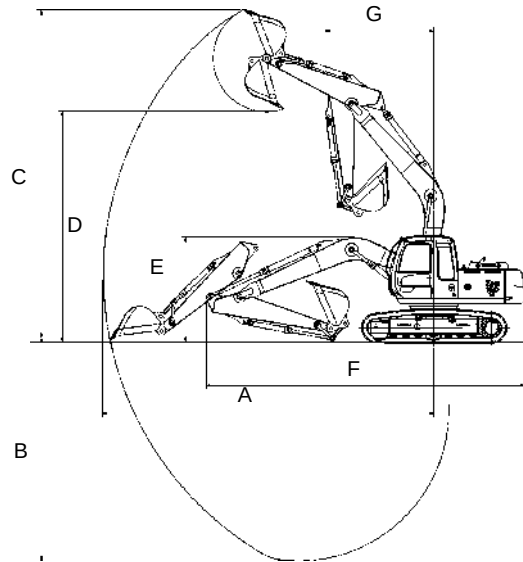
Retroexcavadora
