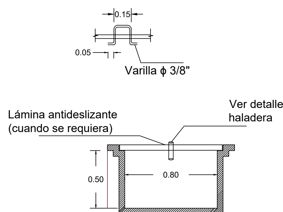
DETALLE CÀRCARMO BT. UNIDADES EN METROS (m). ESCALA 1:20
