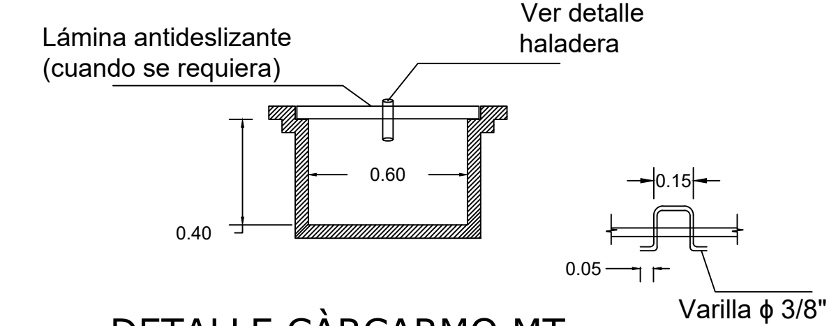
DETALLE CÀRCARMO MT. UNIDADES EN METROS (m). ESCALA 1:20
