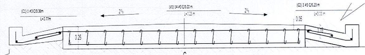
Ilustración 5, Armadura aceros viga transversal Placa Huella con sección de cuneta tipo “L”
