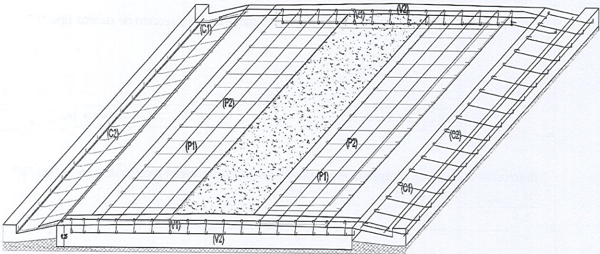
Ilustración 4, Distribución aceros en sección isométrica con sección de cuneta tipo “L”
