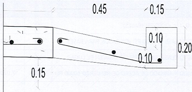
Ilustración 12, Sección transversal de cuneta tipo “L”
