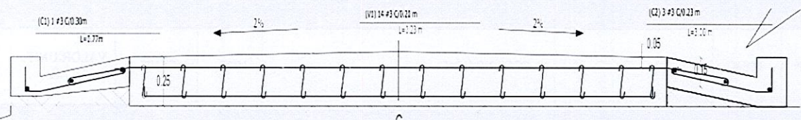
Ilustración 11, Armadura aceros viga transversal Placa Huella sin sobre ancho con sección de cuneta tipo “L”
