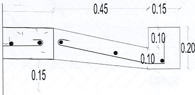
Ilustración 6, Sección transversal de cuneta tipo “L”
