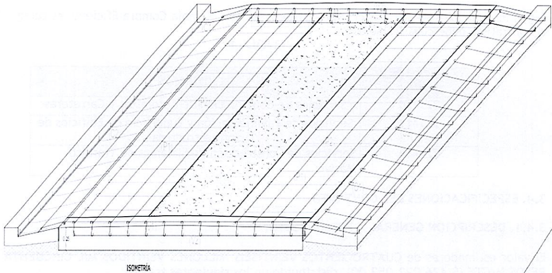
Ilustración 10, Distribución aceros en sección isométrica sin sobre ancho con sección de cuneta tipo “L”
