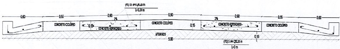
Ilustración 2, Sección Transversal Placa Huella con sección de cuneta tipo “L”
