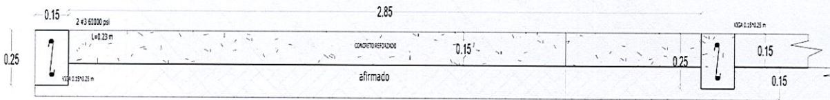
Ilustración 3, Sección longitudinal Placa Huella
