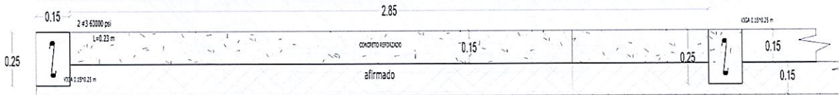
Ilustración 8, Sección Transversal Placa Huella sin sobre ancho con sección de cuneta tipo “L”
