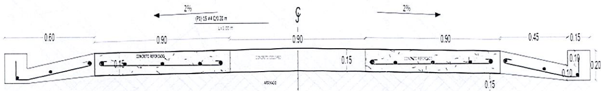
Ilustración 8, Sección Transversal Placa Huella sin sobre ancho con sección de cuneta tipo “L”
