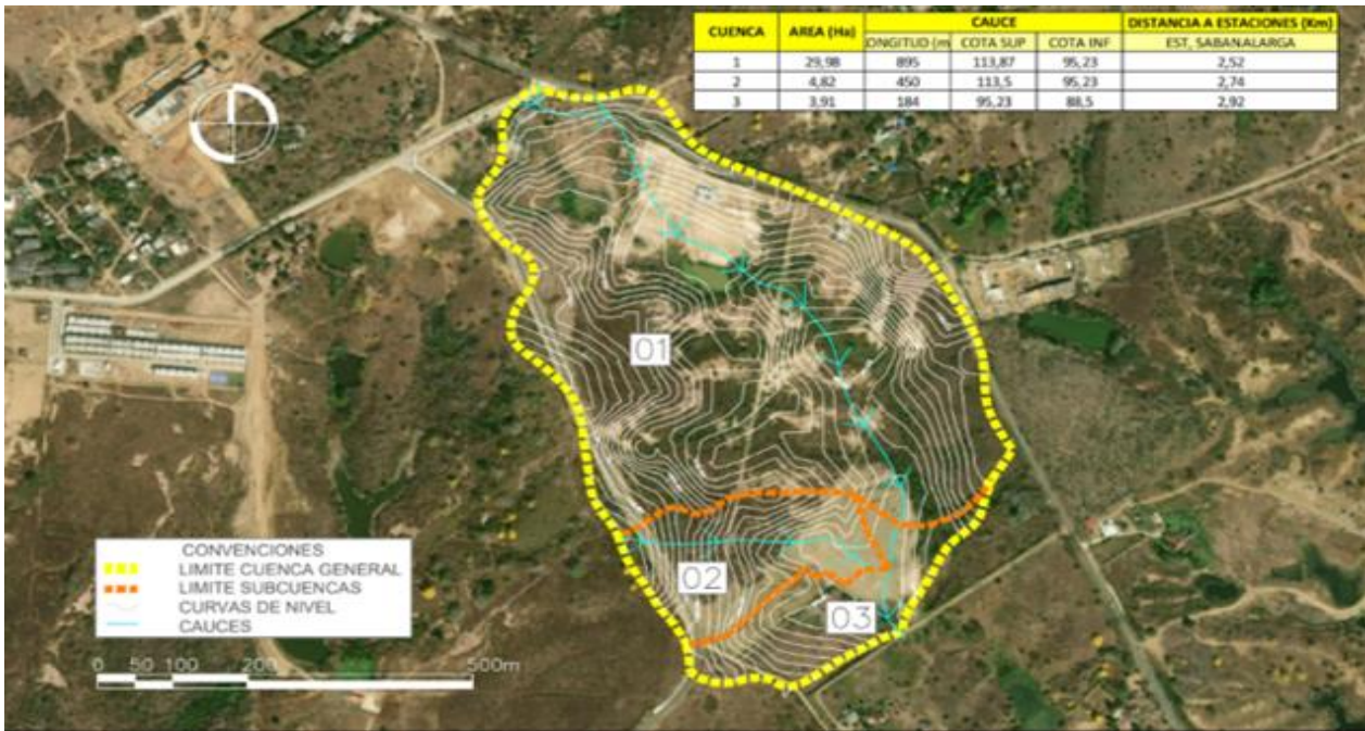
Figura 2. Cuenca general y subcuencas Urbanización Villa Yady Sabanalarga- Atlántico.
