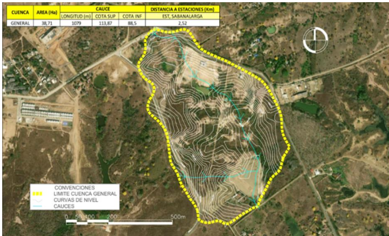
Figura 1. Cuenca General de predio de mayor extensión Urbanización Villa Yady Sabanalarga- Atlántico.
