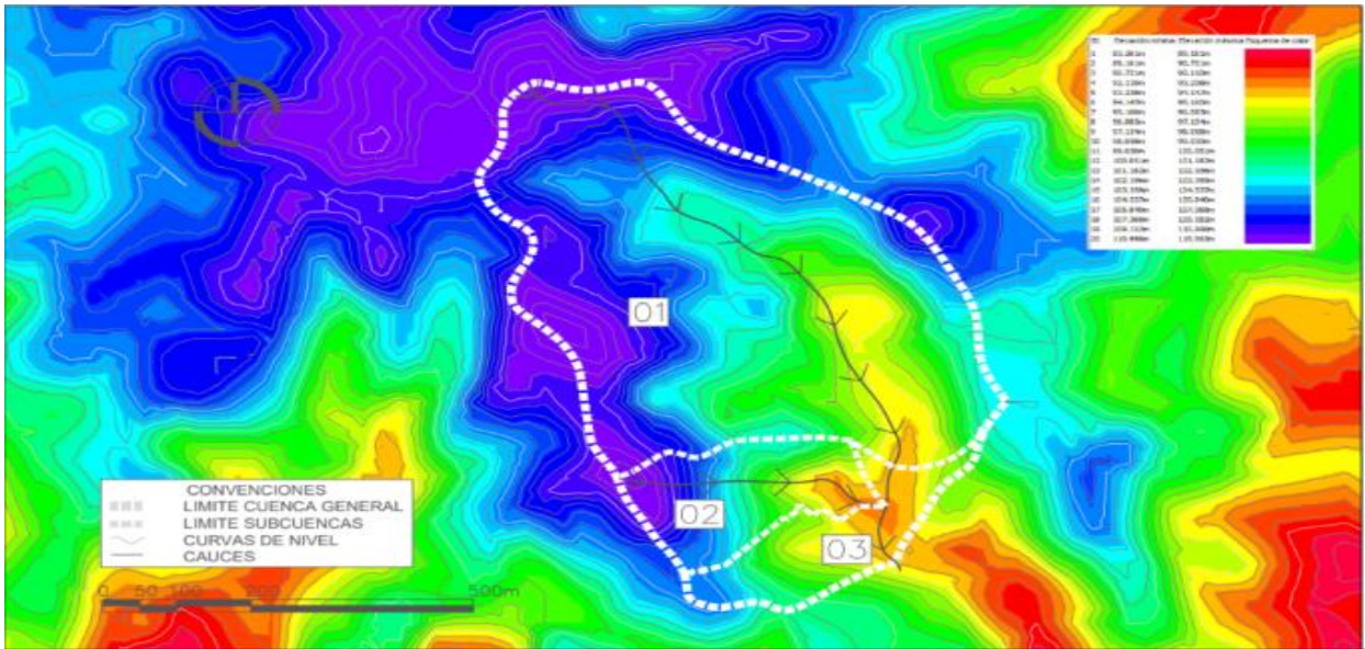
Figura 3. Modelo digital de elevaciones Urbanización Villa Yady Sabanalarga- Atlántico.
