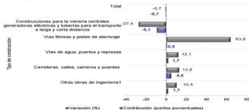
Gráfico 2 IIOC. Variación anual y contribución a la variación de los pagos en obras civiles según tipos de construcción 2016 pr (II trimestre)
