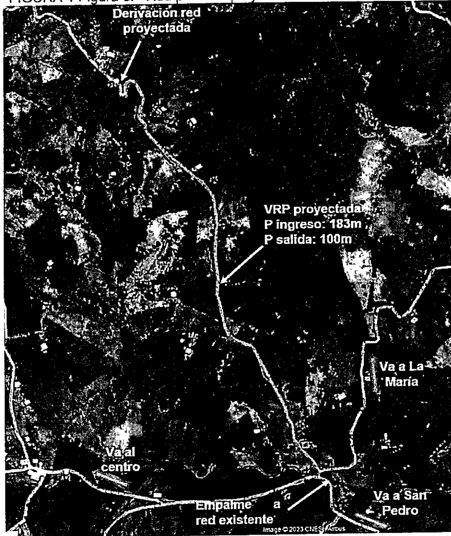
FIGURA 1 Figura 5. Red primaria proyectada PE 100 PN 20 Ø90mm.
