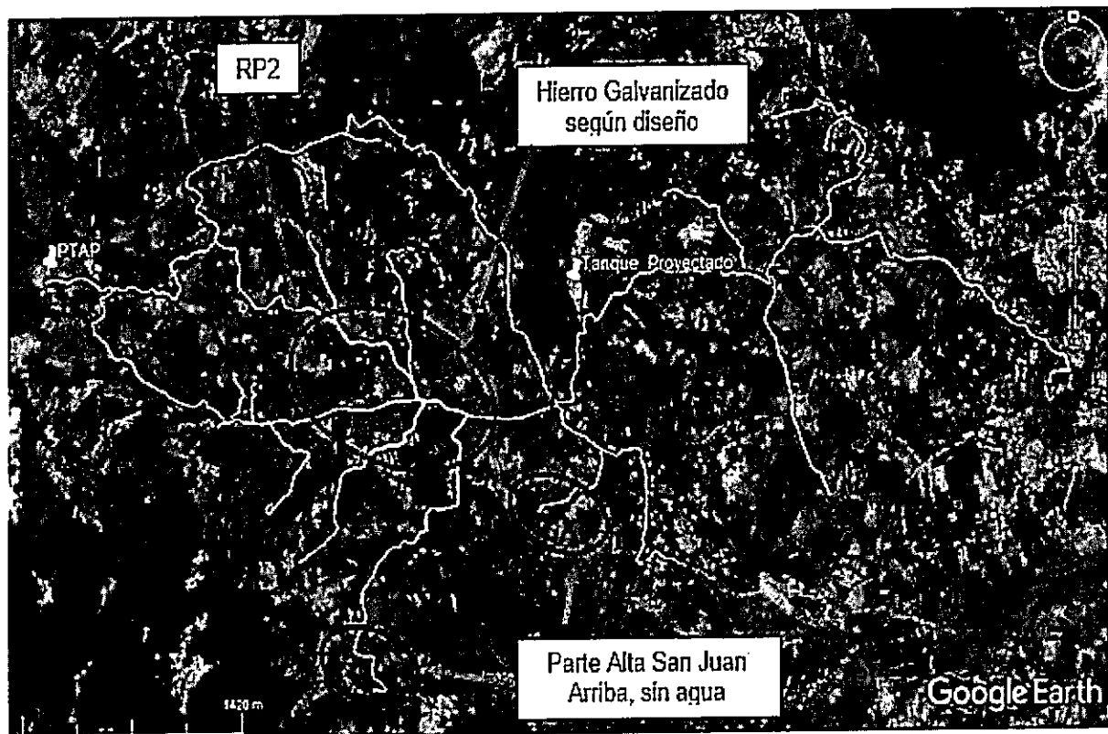
FIGURA 2 RED DE DISTRIBUCIÓN EXISTENTE VEREDA SAN JUAN – LA MARIA
