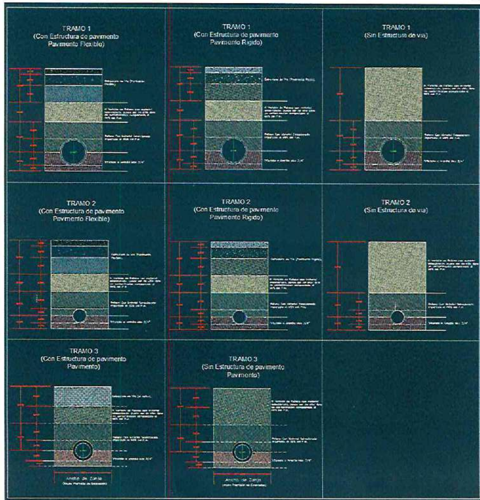
Ilustración 4 Estructura tipo para excavaciones en los tres tramos, la diferencia es el diámetro de la tubería.
