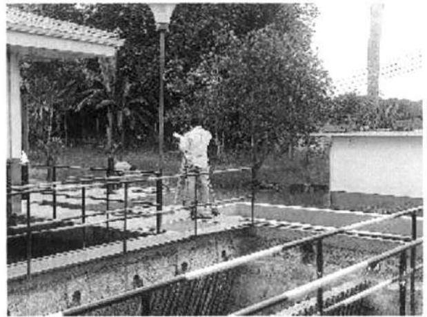
Foto 14. Topógrafo del contratista realizando actividades de nivelación y verificación de medidas con el ingeniero Diego Montoya en la planta de Guacarí
