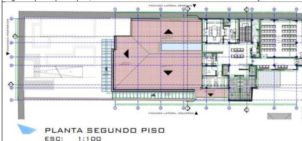
Figura 2. planta segundo piso, nueva sede de la e.s.e centro de salud de Jerico - Boyacá.
