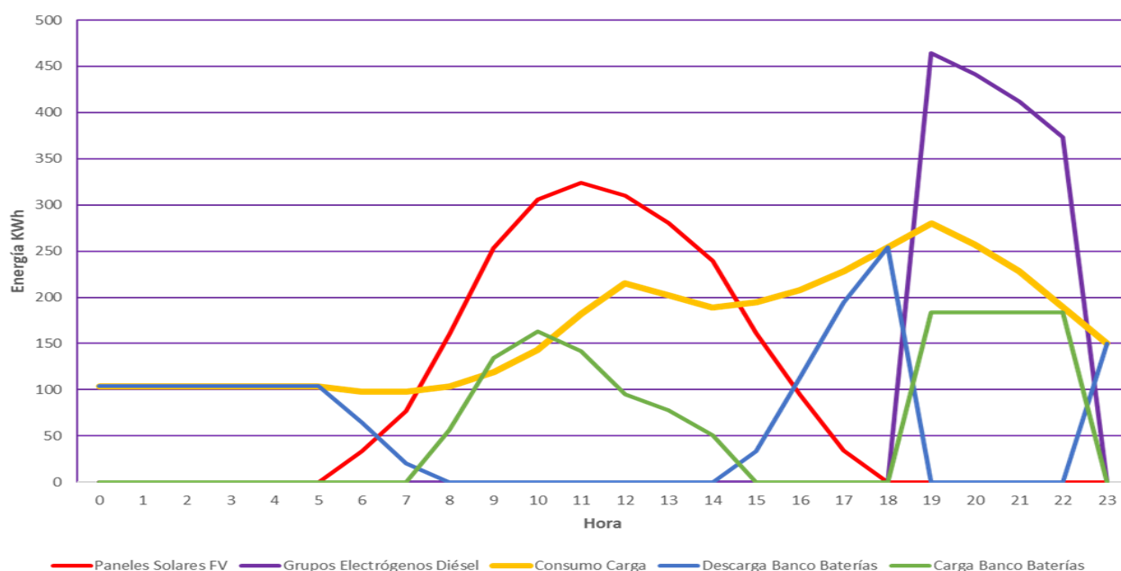
Figura 3: Balance Diario Energía SHSFC-Diesel Isla Grande – Islas del Rosario – Municipio de Cartagena – Departamento de Bolívar
