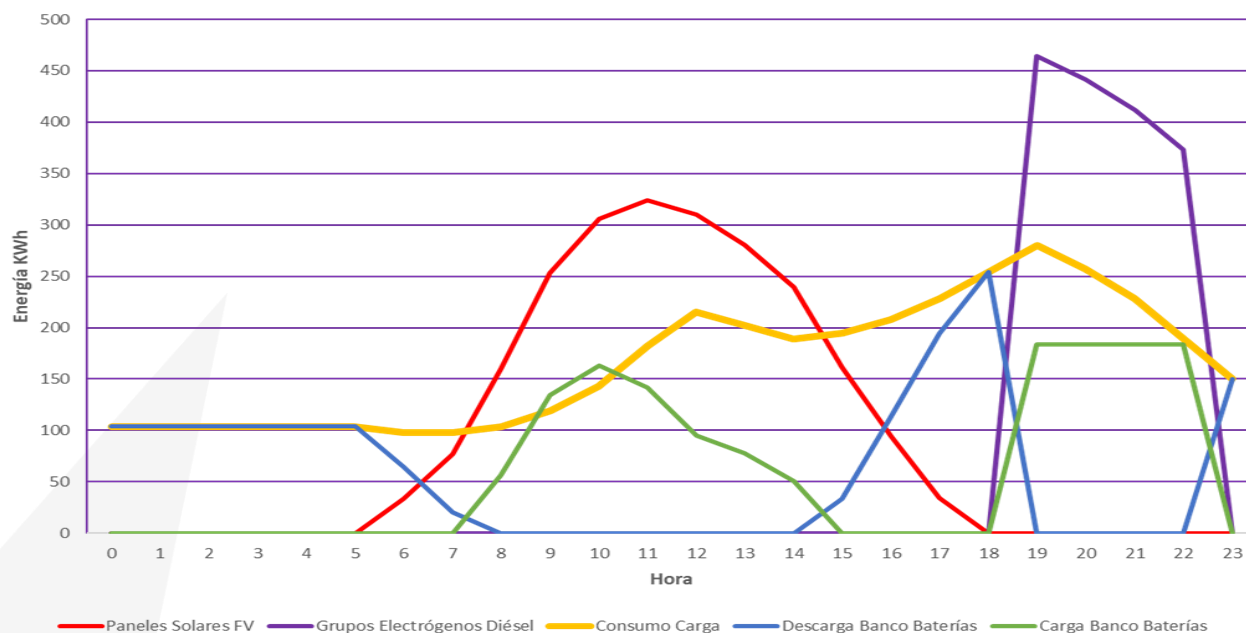
Figura 3: Balance Diario Energía SHSFC-Diesel Isla Grande – Islas del Rosario – Municipio de Cartagena – Departamento de Bolívar
