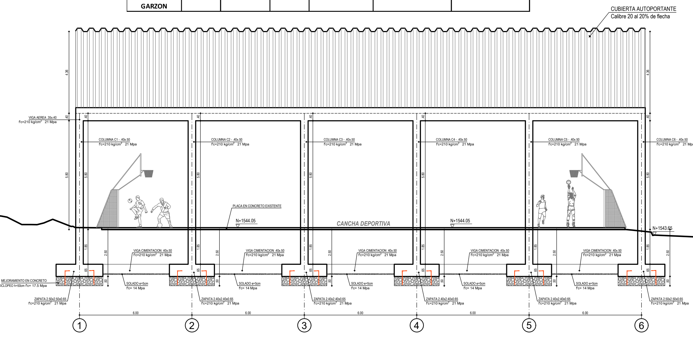
CORTE LONGITUDINAL B-B' ESCALA 1:125
