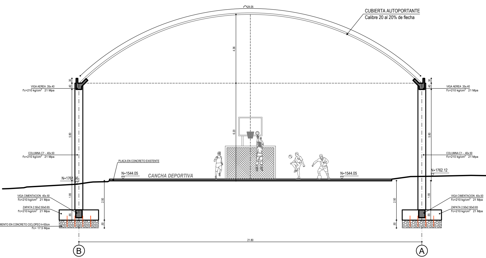
CORTE TRANSVERSAL A-A' ESCALA 1:125
