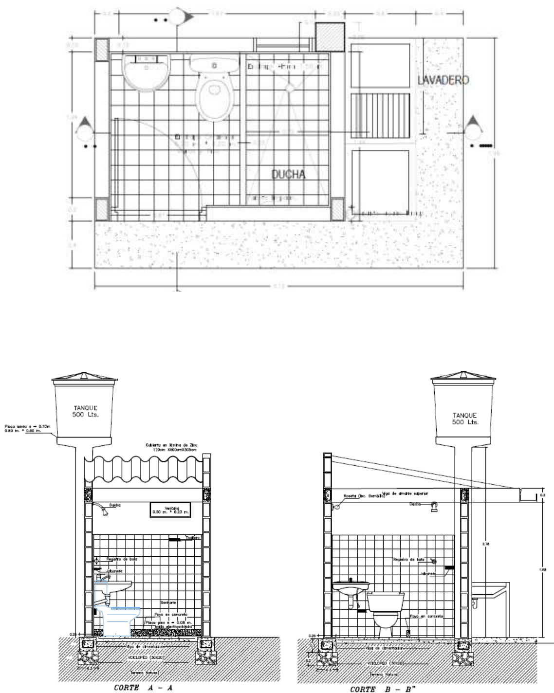
Figura 5: Planos de construcción.
