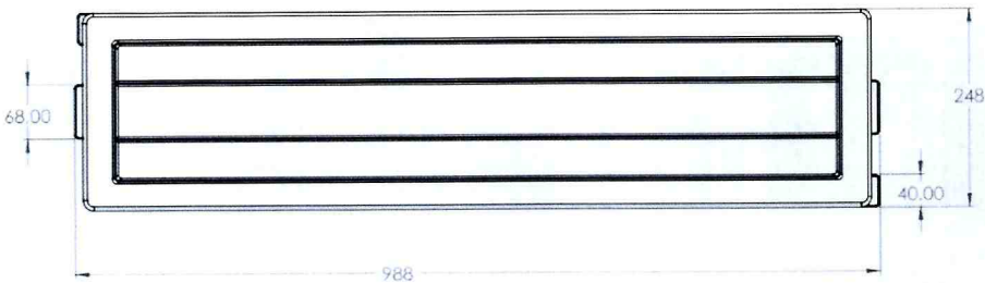
Figura 13. Dimensiones vista superior tapa estándar litoteca nacional (mm)
