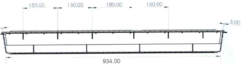
Figura 12. Dimensiones (mm)
