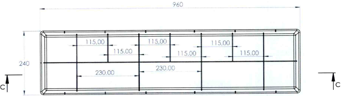
Figura 10. Dimensiones cajas estándar litoteca nacional (mm)
