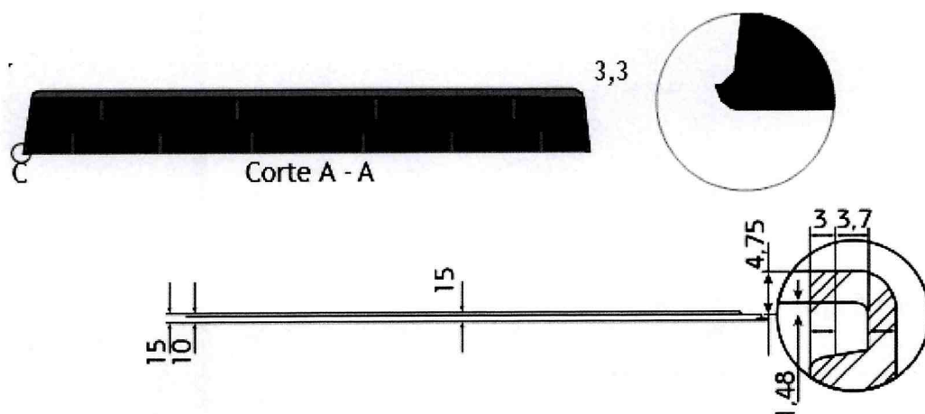
Figura. 9. Ajuste tapa-base medidas en mm.
