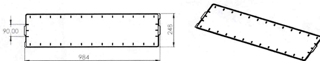
Figura 5. Guías para ajuste TAPA-FONDO (mm)
