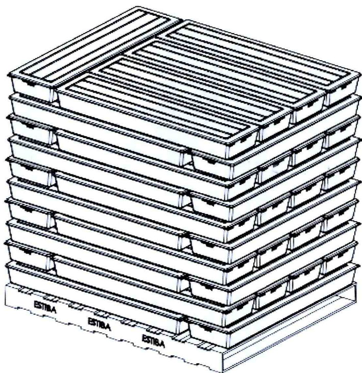
Figura 17. Apilamiento cajas estándar litoteca nacional con máxima capacidad
