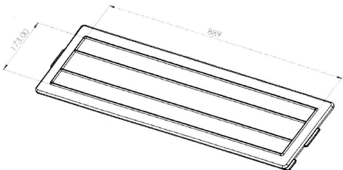
Figura 14. Dimensiones venas de refuerzo tapa estándar litoteca nacional (mm)
