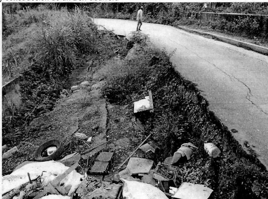
Foto #1. Pérdida de banca K5+200, Cunday – Villarrica.
