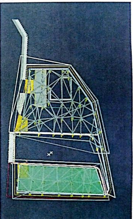
Figura 3: Área donde se realiza relleno con material de subbase. Fuente: Elaboración propia a partir de software Civil 3D.
