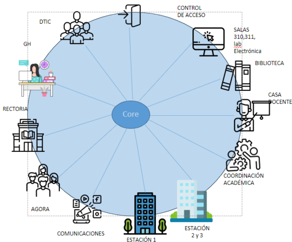
Ilustración 1. Configuración de Red en Sede Avenida Sexta.
