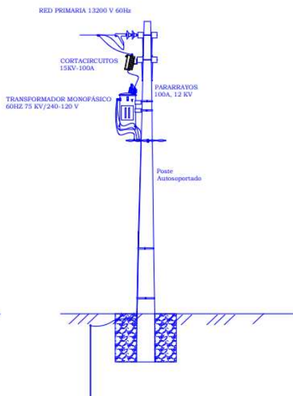
DETALLE ESTRUCTURAS TERMINALES Y ALINIADAS - MONTAJE TRANSFORMADOR-LUMINARIA SOBRE POSTE DE BAJA
