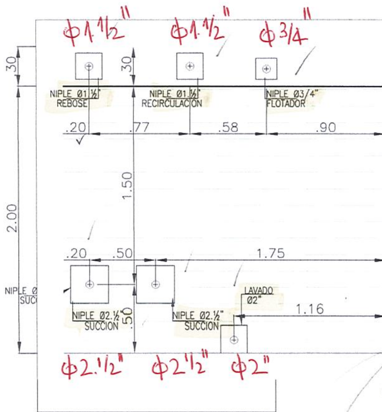
CORTE DE NIPLES N1-N1 AGUA POTABLE ESC 1:25
