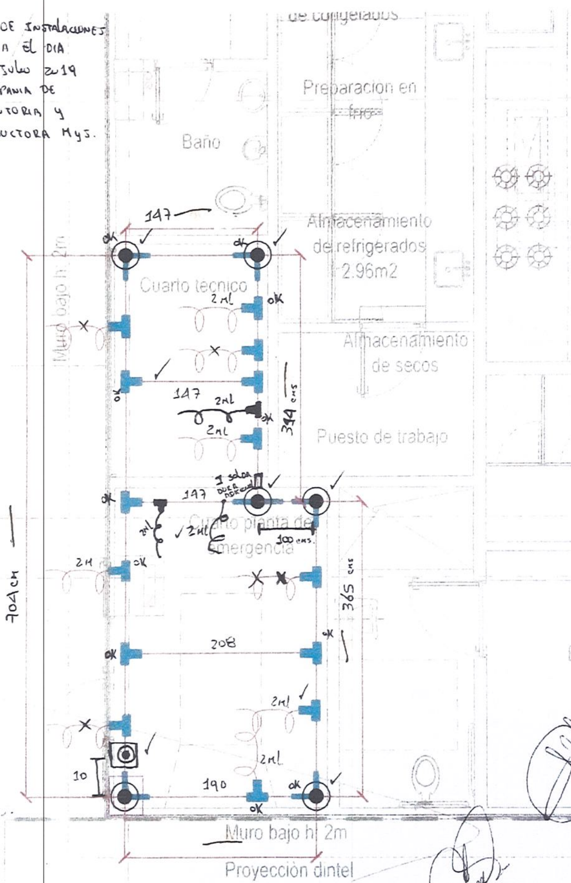
PLANTA DE MALLA DE PUESTA A TIERRA ESC 1:25
