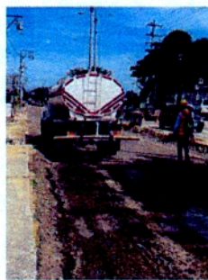
EXTENSIÓN Y HUMECTACIÓN DE MATERIAL DE SUB BASE GRANULAR TIPO INVIAS CON MOTONIVELADORA Y CARROTANQUE
