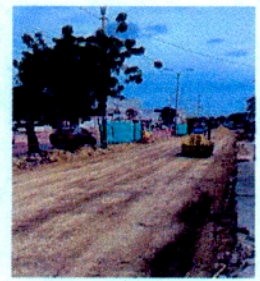
LIMPIEZA Y COMPACTACIÓN DE SUBRASANTE CON EQUIPO MOTONIVELADORA Y VIBROCOMPACTADOR
