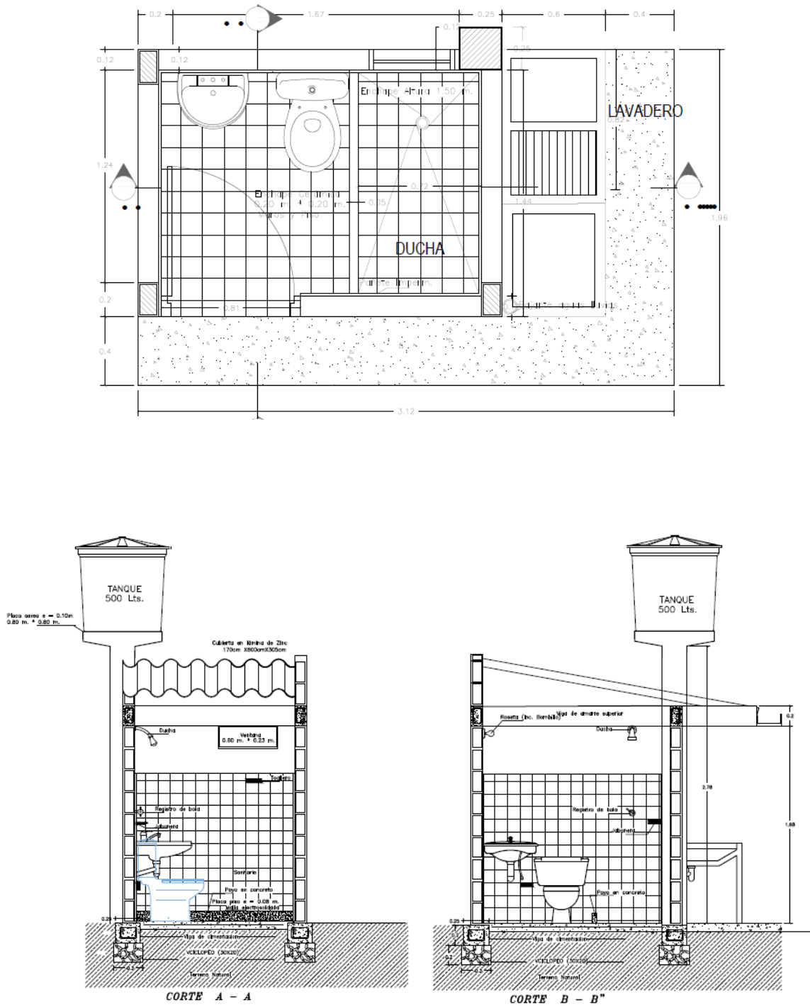
Figura 5: Planos de construcción.
