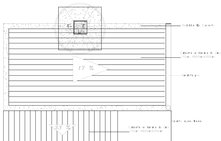
PLANTA CUBIERTA ESCALA 1:15
