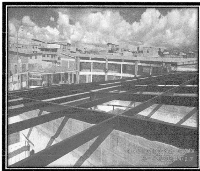
INSTALACIÓN ESTRUCTURA METÁLICA
