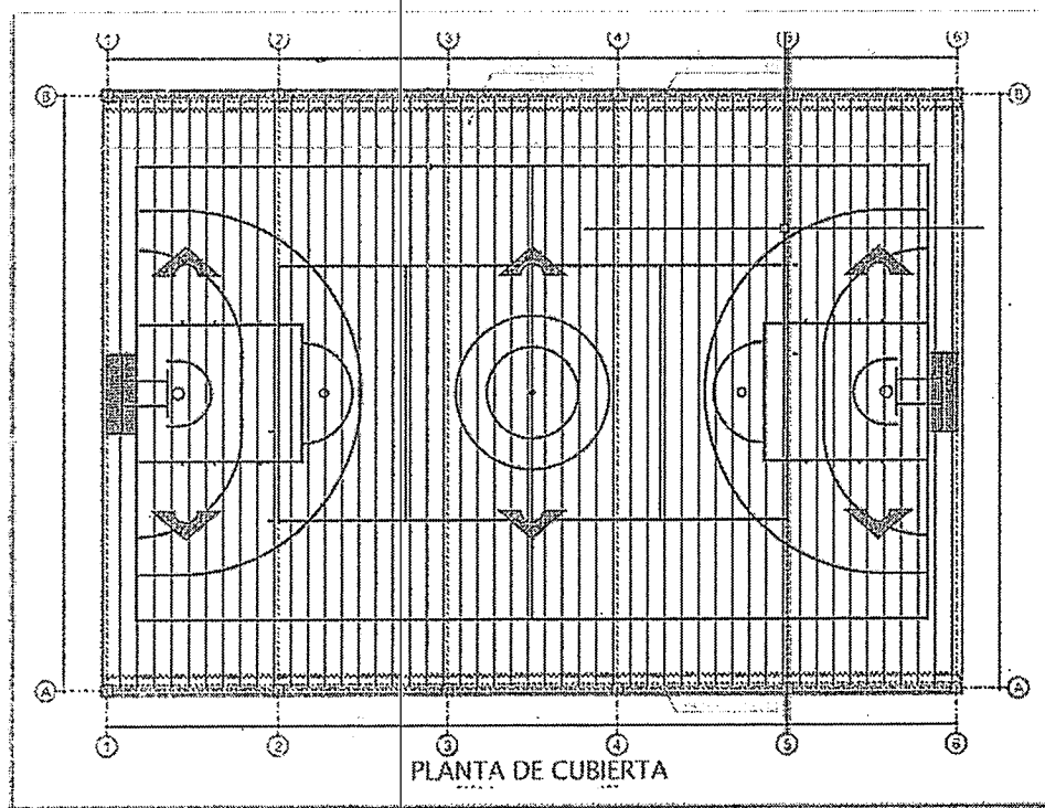
Imagen 3. Planta cubierta.
