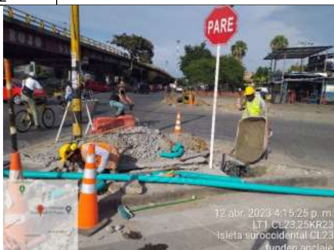
Foto No. 4 | Descripción: Canalización con perforación
