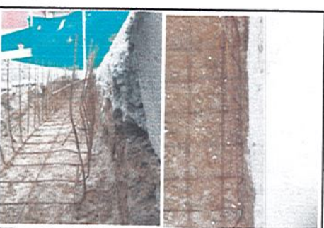
FOTO 8 COLEGIO ALFREDO IRIARTE Refuerzo Caracamo
