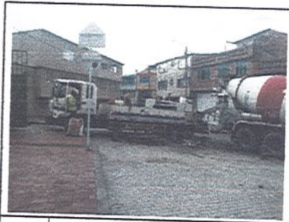
FOTO 15 COLEGIO ALFREDO IRIARTE Concreto y bomba
