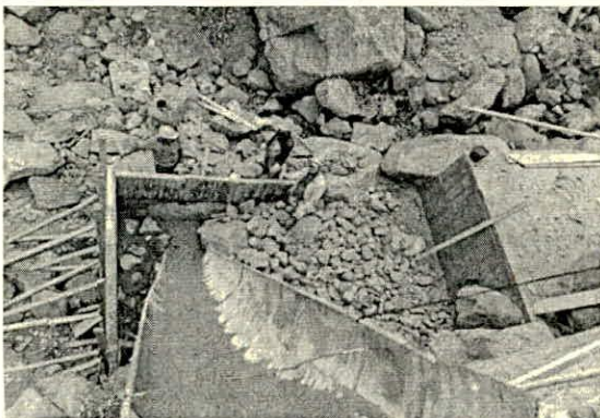
Foto 2: Proceso de fundición de refuerzo en concreto ciclópeo.
