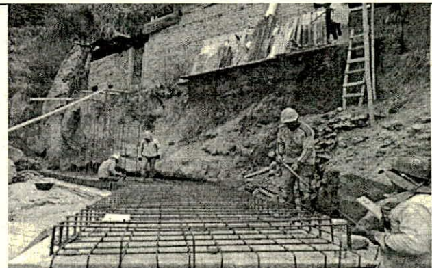
Foto 3: Armado de acero para fundición de zarpa.
