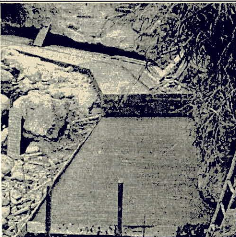
Foto 6: Fundición de refuerzo en concreto ciclópeo PR0+130.
