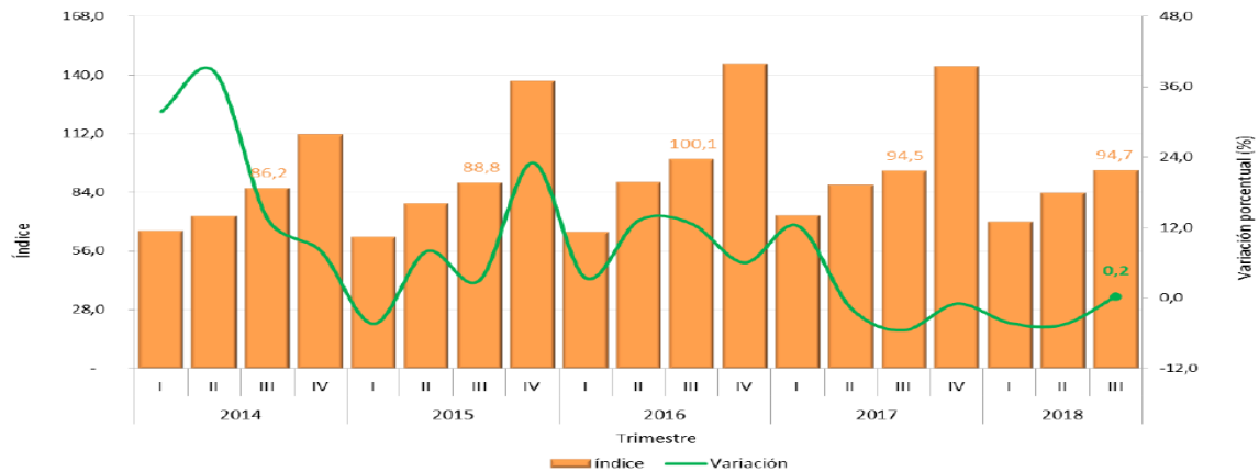
Gráfico 6. Índice y variación anual de los pagos de carreteras, calles, caminos, puentes, carreteras sobreelevadas, túneles y construcción de subterráneos Total nacional – serie empalmada 2014 (I trimestre) – 2018 pr (III trimestre)
