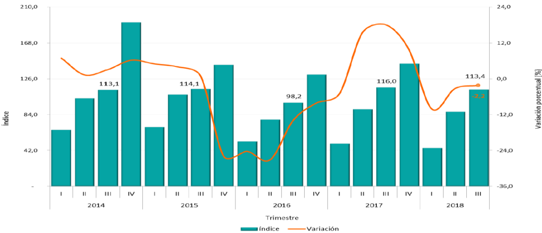
Gráfico 4. Índice y variación anual de los pagos de construcciones para la minería, centrales generadoras eléctricas y tuberías para el transporte a larga y corta distancia Total nacional – serie empalmada 2014 (I trimestre) - 2018 Pr (III trimestre)
