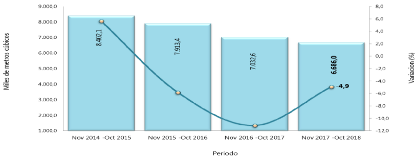
Gráfico 4. Producción y variación de Concreto premezclado en periodos acumulados doce meses (miles de metros cúbicos y variación porcentual) Total nacional 2014 (Noviembre) - 2018 p (octubre)
