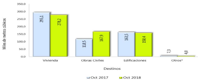
Gráfico 1. Producción de concreto premezclado según destinos (Miles de metros cúbicos) Total nacional Octubre (2017 - 2018) P
