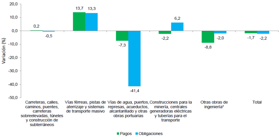
Gráfico 1. Variación anual de los pagos y obligaciones en obras civiles según tipo de construcción Total nacional III trimestre 2018 pr
