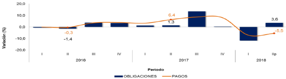
Gráfico 19. Variación anual del IIOC de los pagos y obligaciones en obras civiles (serie empalmada) 2016 (I trimestre) – 2018 (II trimestre) P
