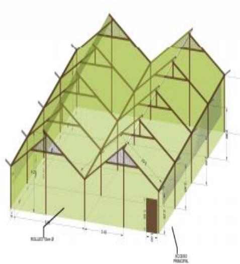
Plano Isométrico.
