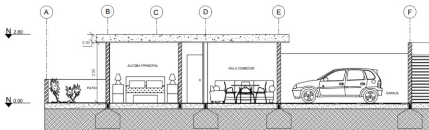
CORTE LONGITUDINAL B-B' Esc:1:50
