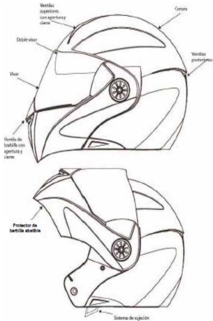
Figura ilustrativa 2. Casco de Seguridad para Motociclista Tipo "2" Abatible o Escualizable
