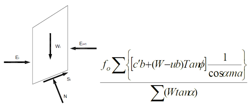
Figura 29. Método Jambu
