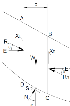
Figura 30. Método Spencer
