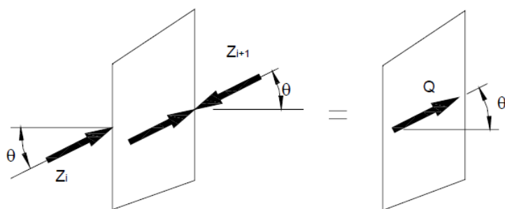
Figura 31. Método Morgenstern and Price
