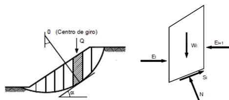
Figura 27 Tajadas en una ladera y Diagramas de fuerzas analizadas pro Bishop
