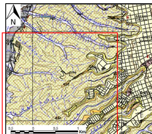
Figura 3. Formación Bucaramanga Miembro Órganos (Qbo), al oeste del Municipio de Bucaramanga (Tomado de INGEOMINAS, 2001).
