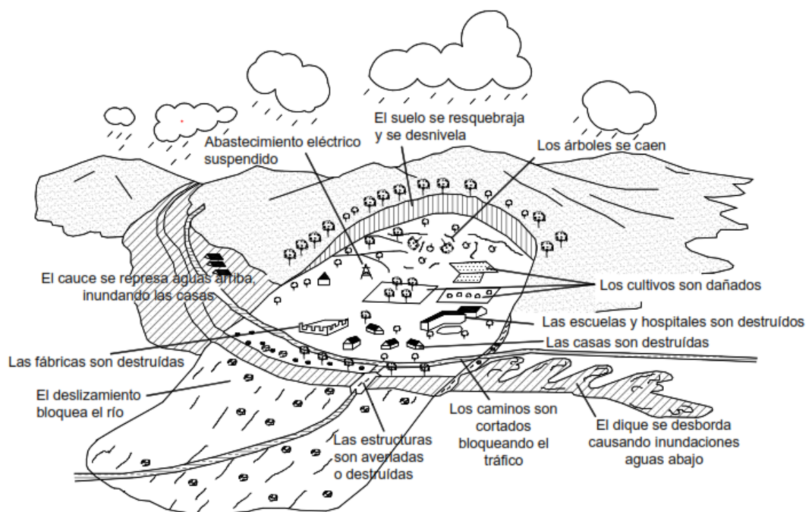
Figura 12. Deslizamiento sobre zona poblada
