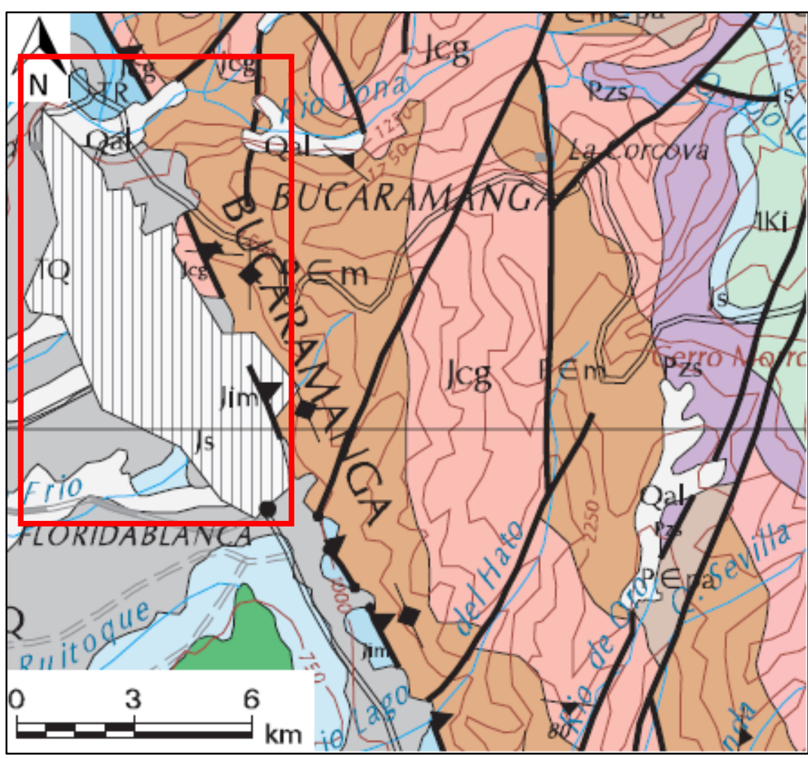
Figura 1. Unidad Neis de Bucaramanga ubicada al este del Municipio de Bucaramanga (Tomado de INGEOMINAS, 1999).
