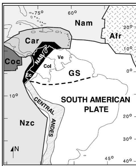
Figura 8. Bloque Norandino en la esquina septentrional de Suramérica y su compleja interacción con las Placas Nazca, Caribe y Suramérica. Tomado de Cediel et al., 2003.
