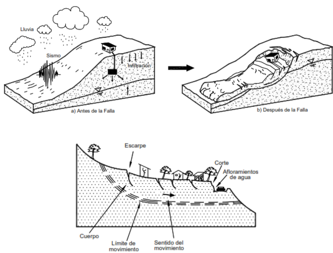
Figura 16. Deslizamiento en suelos blandos
