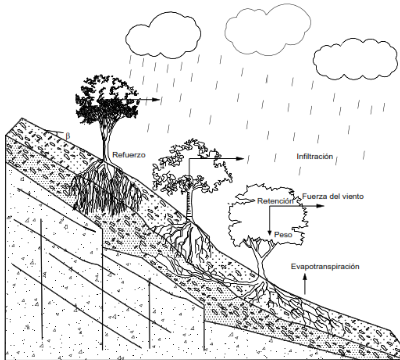
Figura 23. Refuerzo de taludes con vegetación
