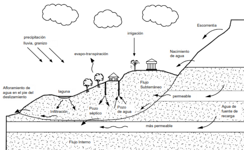
Figura 18. Infiltración del agua en laderas
