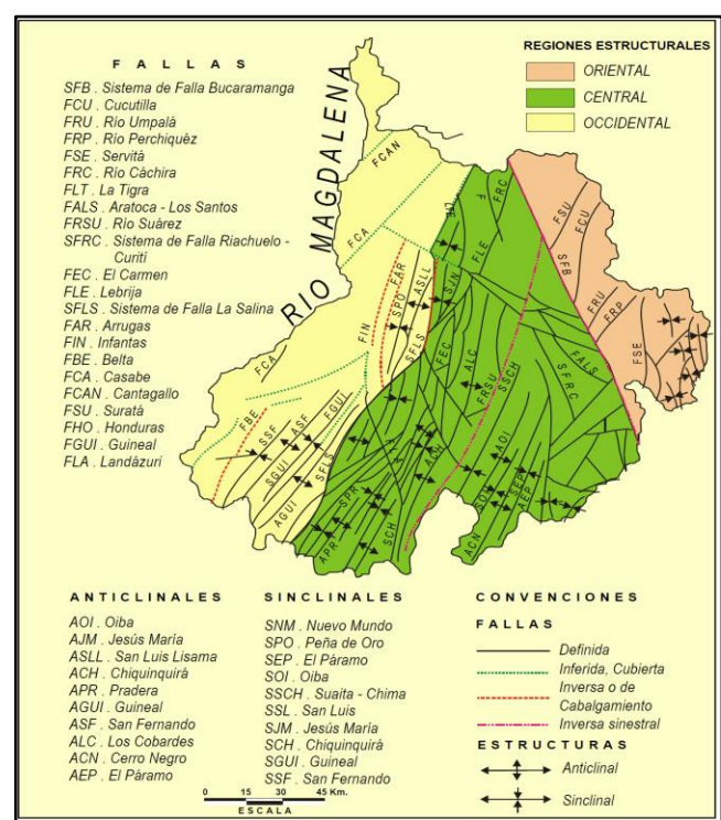
Figura 10. Esquema estructural del Departamento de Santander. Tomado de Royero y Clavijo, 2001.
