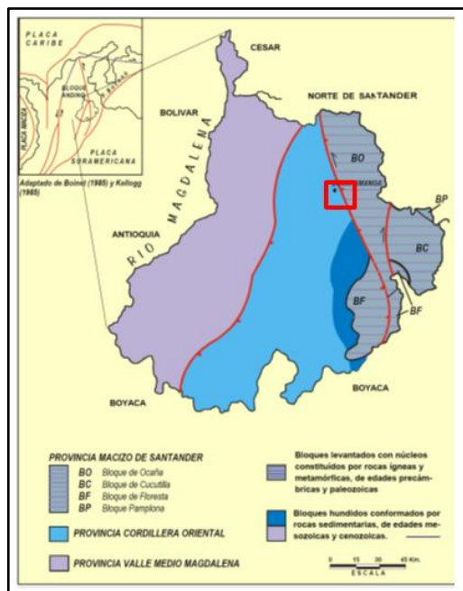
Figura 9. Esquema tectónico del Departamento de Santander. En el cuadro rojo se encuentra el área de estudio. Modificado de Royero y Clavijo, 2001.
