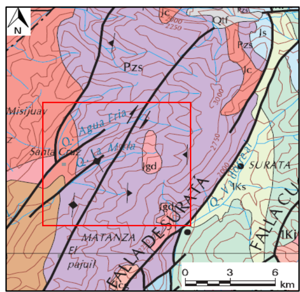
Figura 2. Formación Silgará en los alrededores de Matanza y Surata. Ubicada al Noreste del Municipio de Bucaramanga (Tomado de INGEOMINAS, 1999).
