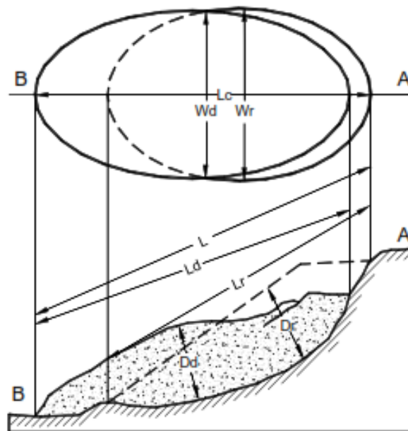
Figura 15. Dimensiones de los movimientos en masa IAEG Commission on Landslides (1990).
