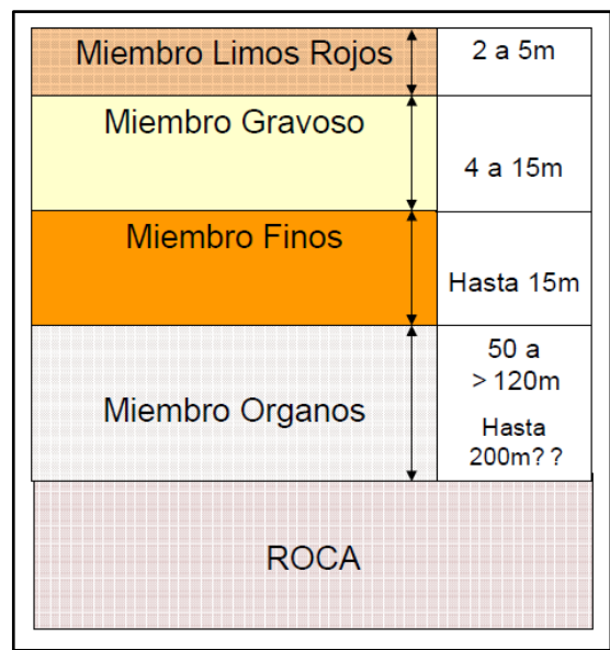
Figura 7. Perfil típico y espesores promedio de la Formación Bucaramanga (Tomado de INGEOMINAS, 2001).
