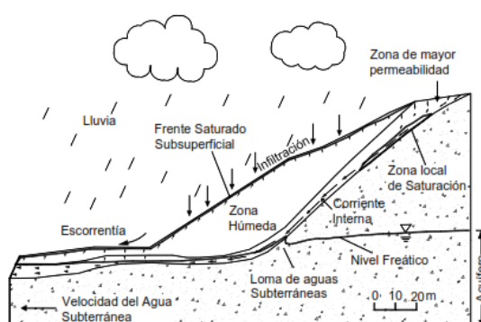
Figura 17. Esquema de precipitación e infiltración.
