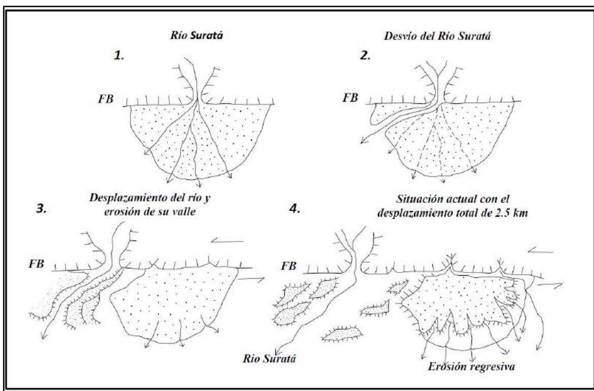
Figura 11. Desvío del Río Suratá debido a la acción de la Falla de Bucaramanga. Tomado de Diederix et al., 2008.
