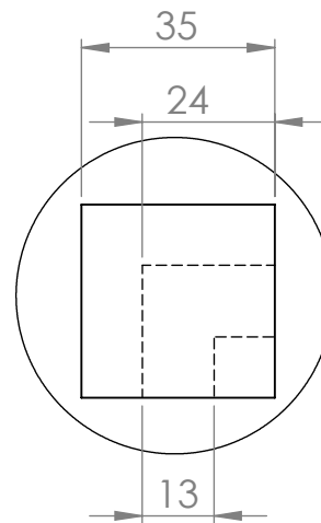
DETALLE A ESCALA 2 : 3
