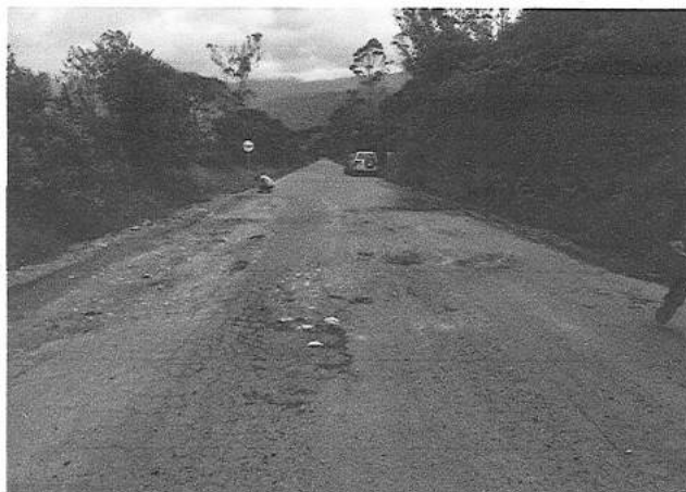
PR 22+760
