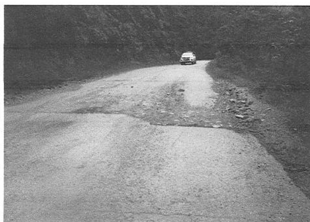
PR 5+420
