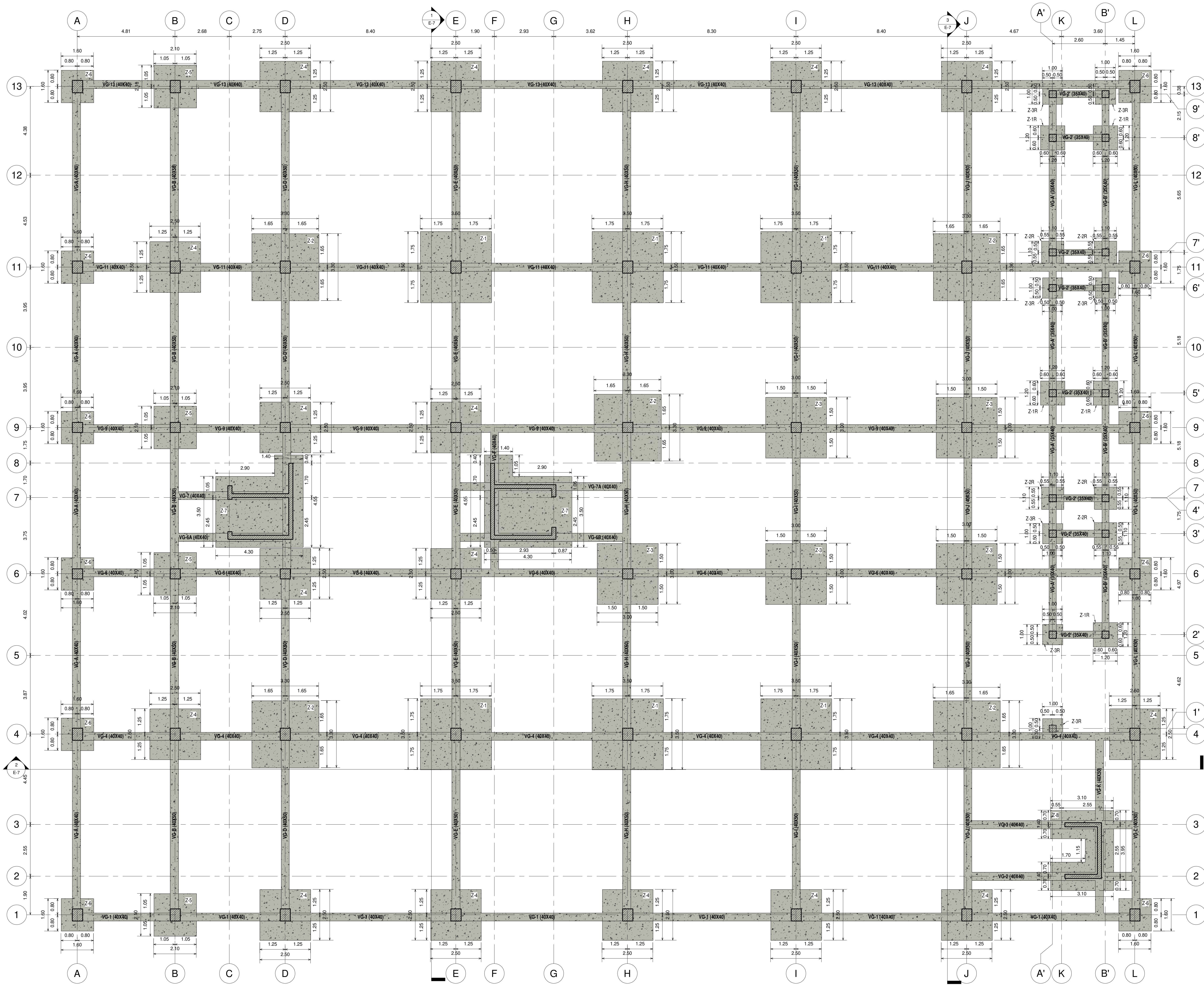
PLANTA DE CIMENTACION N-1.50 ESC. 1:75
