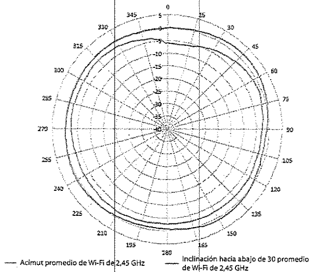
Wi-Fi de 2,45 GHz (antenas 1, 2)
