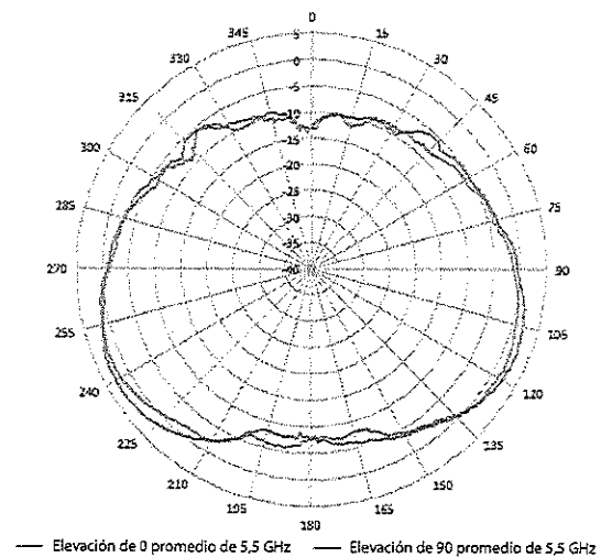
Wi-Fi de 5,5 GHz (antenas 1, 2, 3, 4)
