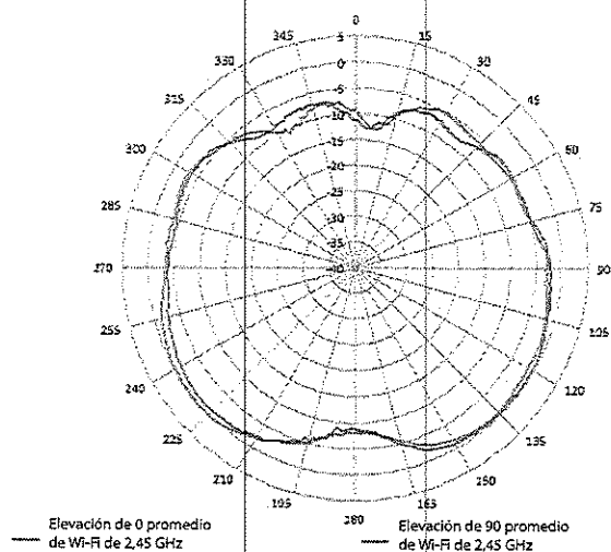
Wi-Fi de 2,45 GHz (antenas 1, 2)
