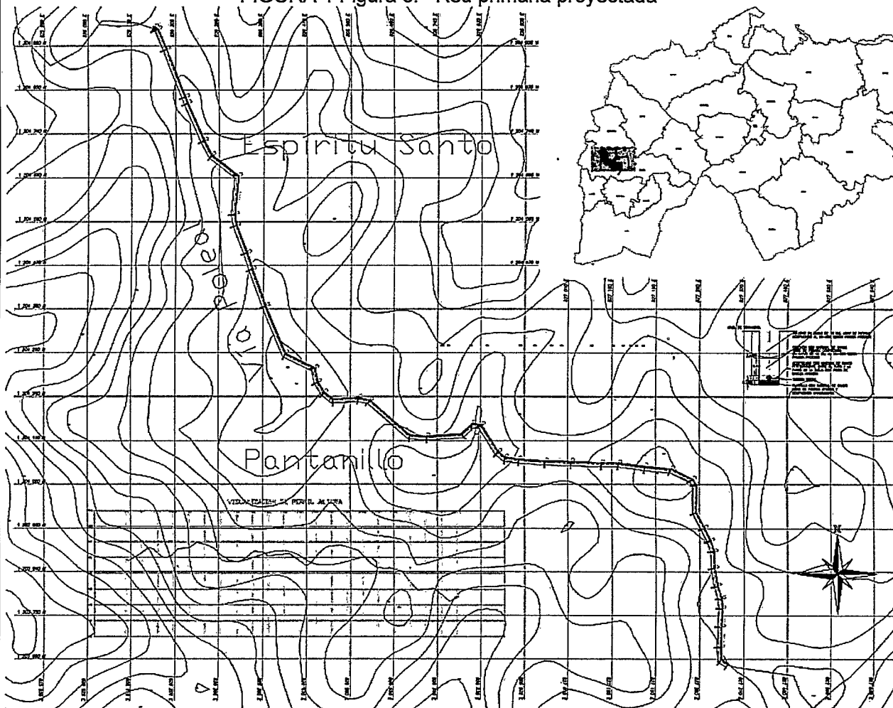
FIGURA 1 Figura 5. Red primaria proyectada
