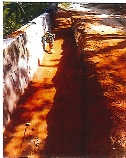
FOTO 6. RELLENO ALCANTARILLA No. 1
