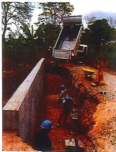
FOTO 9. RELLENO MURO No. 2
