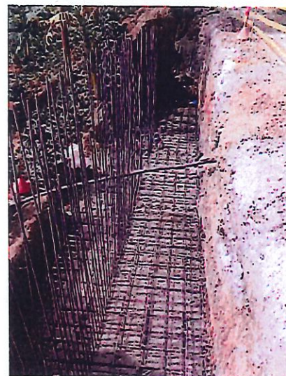
FOTO 19-20 INSTALACIÓN ACERO FIGURADO ALCANTARILLADO No. 1
