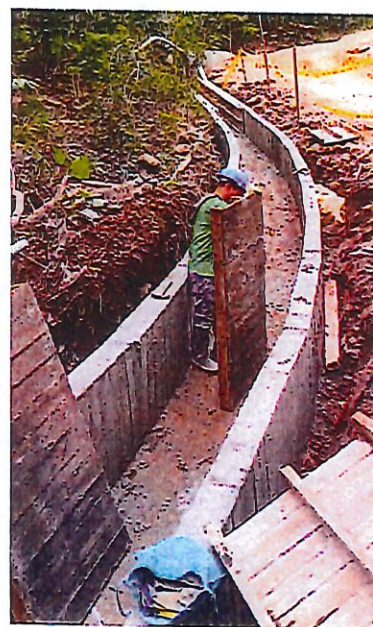
FOTO 16. FUNDICIÓN CANAL ALCANTARILLA No. 3
