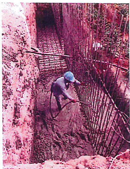
FOTO 21-22 FUNDICIÓN ESTRUCTURA BASE ALCANTARILLA No.1
