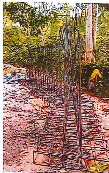
FOTO 12. FIGURACIÓN ACERO ENCOLE ALCANTARILLA No. 3
