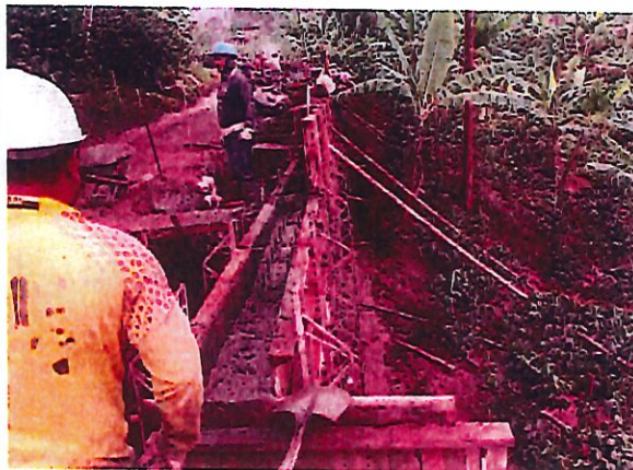
FOTO 28 FUNDICIÓN ESTRUCTURA ELEVADA MURO ALCANTARILLADO No. 1
