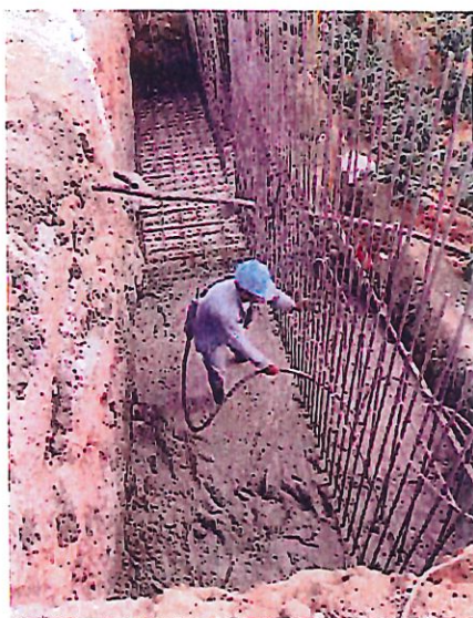
FOTO 21-22 FUNDICIÓN ESTRUCTURA BASE ALCANTARILLA No.1
