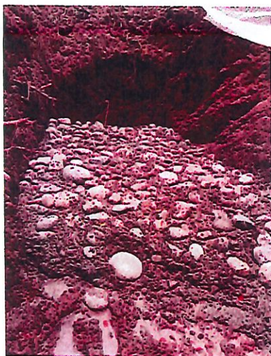
FOTO 15-16 FUNDICIÓN MEJORAMIENTO CICLOPEO ALCANTARILLADO No. 2
