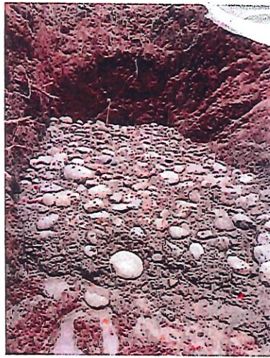
FOTO 15-16 FUNDICIÓN MEJORAMIENTO CICPLOPEO ALCANTARILLADO No. 2
