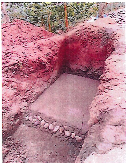
FOTO 13-14 FUNDICIÓN MEJORAMIENTO CICPLOPEO MURO No. 1
