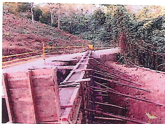
FOTO 31-32. FUNDICIÓN ESTRUCTURA ELEVADA POCETA MURO No. 1
