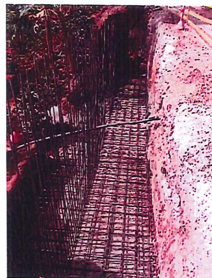
FOTO 19-20 INSTALACIÓN ACERO FIGURADO ALCANTARILLADO No. 1
