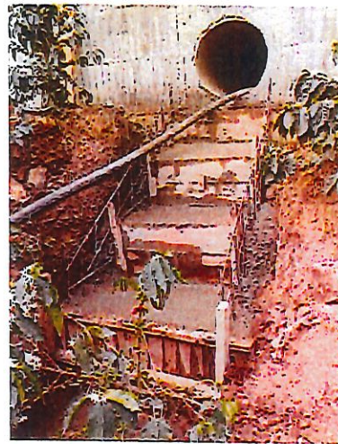
FOTO 10. FUNDICIÓN DISIPADOR ALCANTARILLA No. 1
