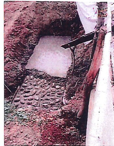
FOTO 15-16 FUNDICIÓN MEJORAMIENTO CICPLOPEO ALCANTARILLADO No. 2
