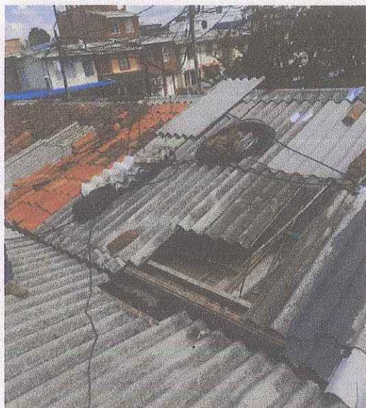
Ejecución: Suministro e instalación de teja de fibrocemento perfil 7 (No.8)
