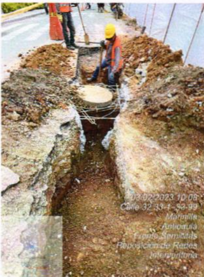
Imagen No.7 F. semillitas_nicho de inspección Valvula de 10"
