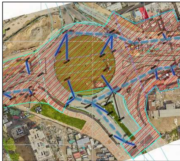
Ilustración 1: Redes de alcantarillado proyectadas en la glorieta Av. Bosa. Fuente: Elaboración propia.
