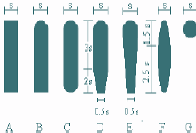
Ilustración 4. Diferentes formas de rejillas
