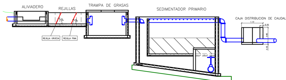
Ilustración 3. Diseño conceptual PTAR proyectada. Fuente: Grupo Consultor
