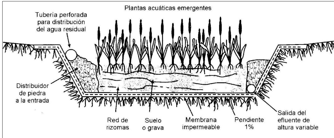
Figura 3. Esquema Humedal Artificial o Biofiltro
