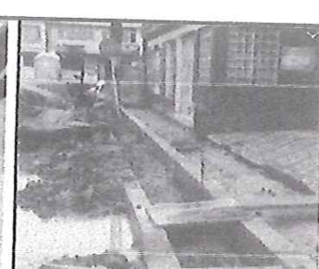
Instalación de bordillo y figurado de hierro para fundida de andenes CIV 16003173
