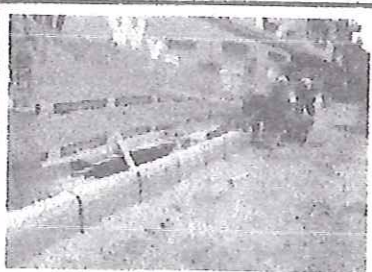
Instalación de sardinel prefabricado tipo A-10 costado occidental
