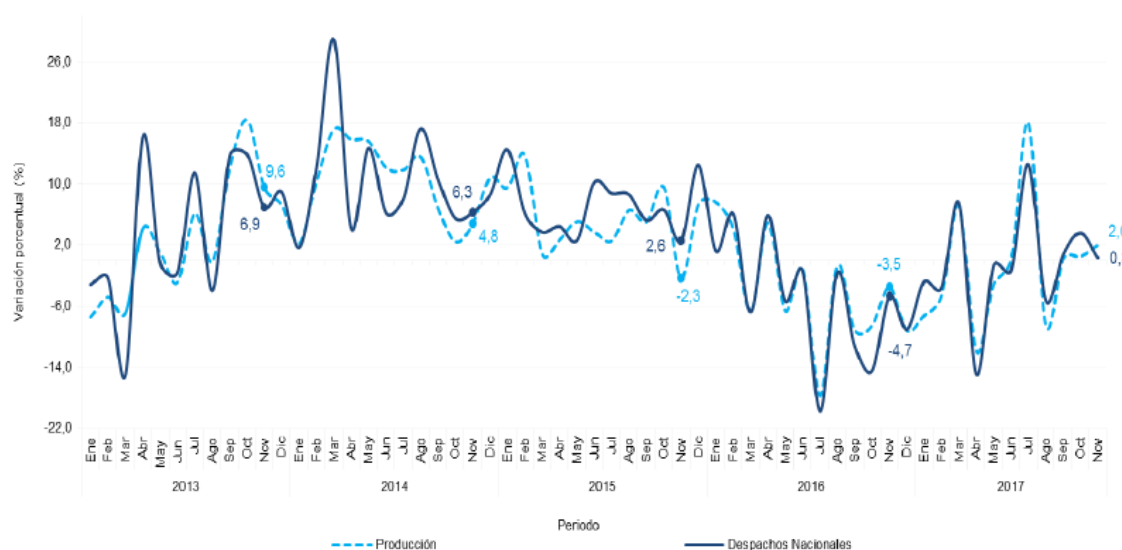
Gráfico 2. Variación anual de la producción y los despachos nacionales de cemento gris Total nacional 2013 (enero) – 2017 (noviembre p )
