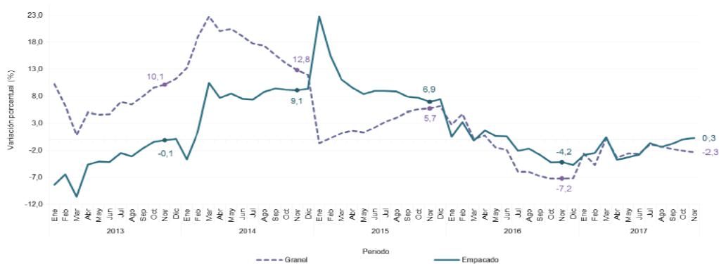
Gráfico 21. Variación año corrido de los despachos nacionales de cemento gris, según tipo de empaque
