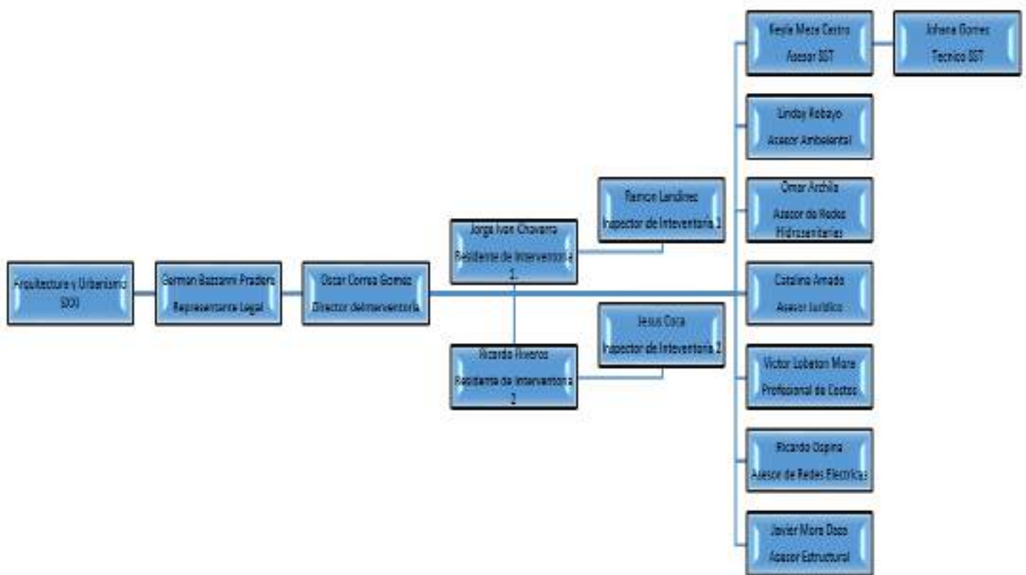
IMAGEN 2 – ORGANIGRAMA INTERVENTORIA.
