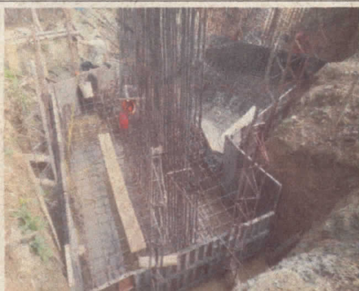
Encofrado para Fundida de Zapatas en Concreto 4000 PSI
